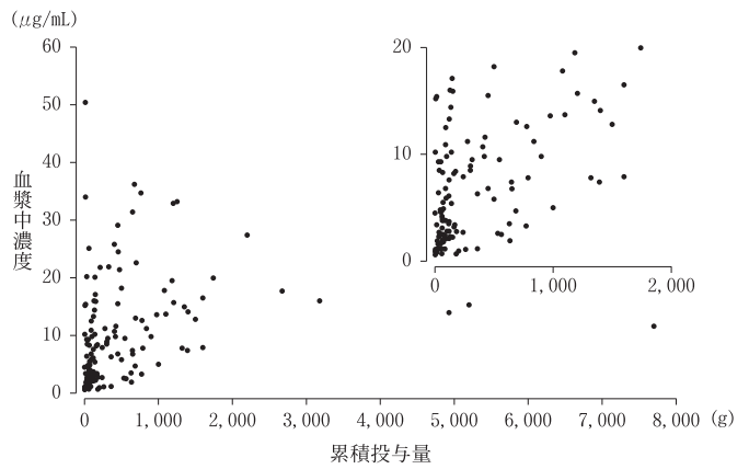
図 本剤の血漿中濃度と累積投与量
